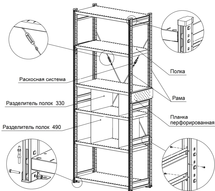
Схема вариантов установки стеллажа СТ-031
