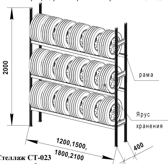
Стеллаж СТ-023 для автомобильных дисков
