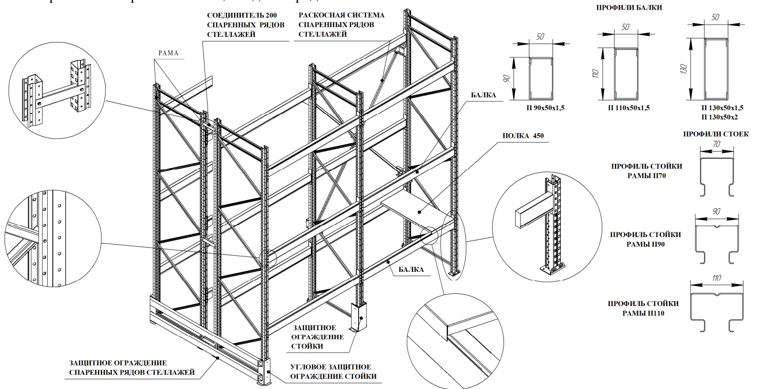
Схема сборки палетных стеллажей
